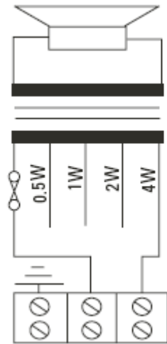
↳ Bekötési rajz
