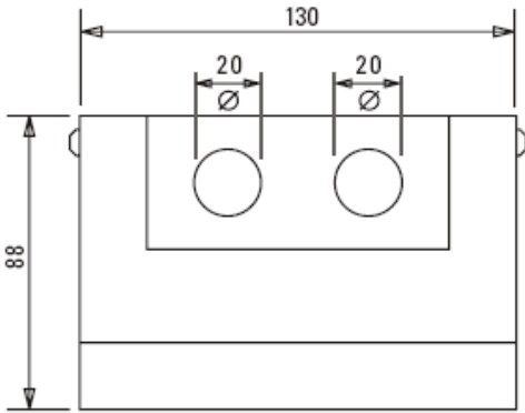
↳ Felülnézet RCS8/T / minden méret mm/
